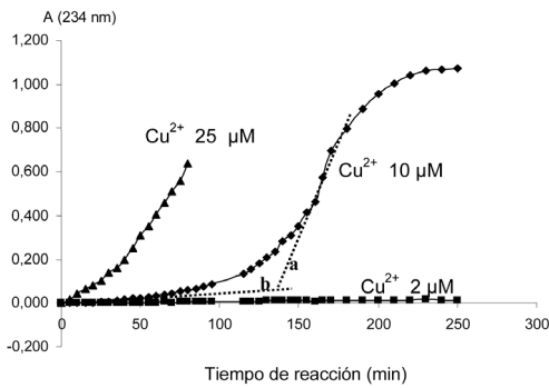
Figura 1.- Efecto de la concentración del Cu 2+ en la cinética de la peroxidación de los ácidos grasos poliinsaturados de la HDL.
