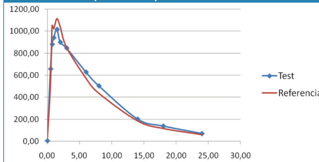
Gráfico N° 1: Comportamiento plasmático de la Levofloxacin
